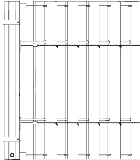
Obr. 2 - boční vedení v lanku
