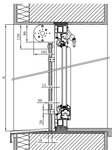
Montáž na stěnu - svislý řez - lišty, průchodka
