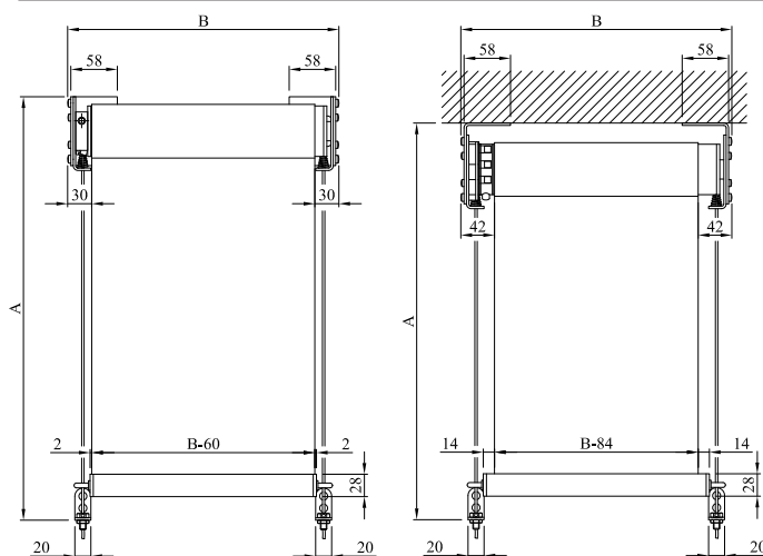
Montáž na stěnu - ruční ovládání
