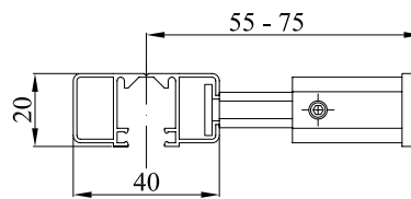
Samonosný systém – vertikální řez
