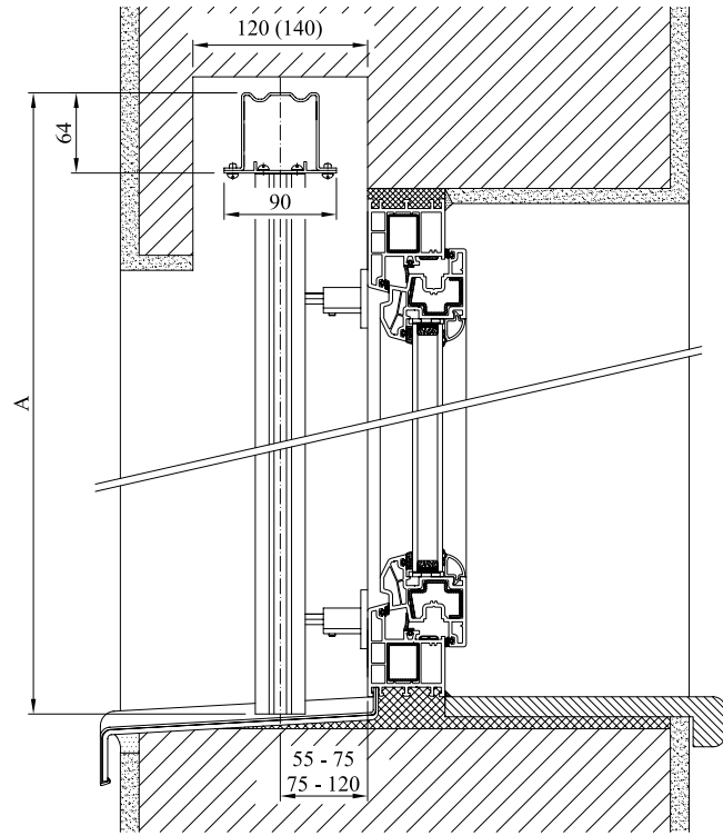
Samonosný systém – vertikální řez
